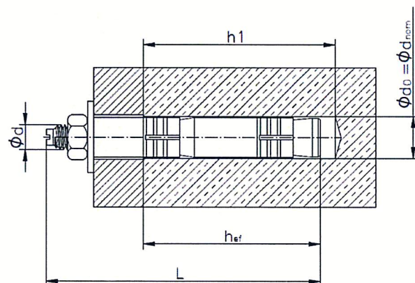
Rysunek B2. Parametry montażu łączników rozporowych SLD
