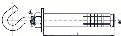
Rysunek A3. Stalowy łącznik jednorozporowy SLC
