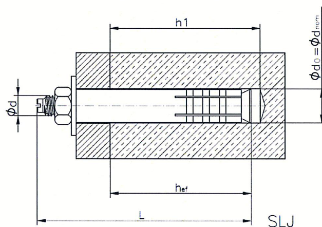
Rysunek B1. Parametry montażu łączników rozporowych SLJ, SLL, SLC i SLO
