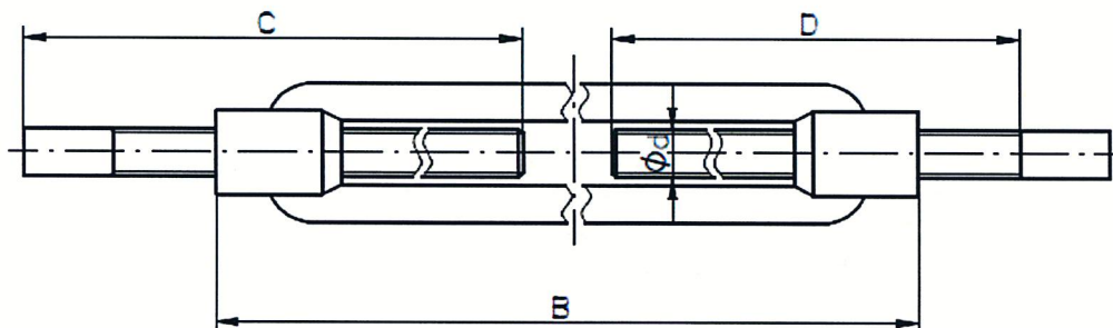
Rys. A3. Łącznik śrubowy dwustronny SRM-HO
