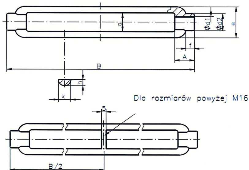
Rys. A5. Łącznik śrubowy dwustronny SRM-OO
