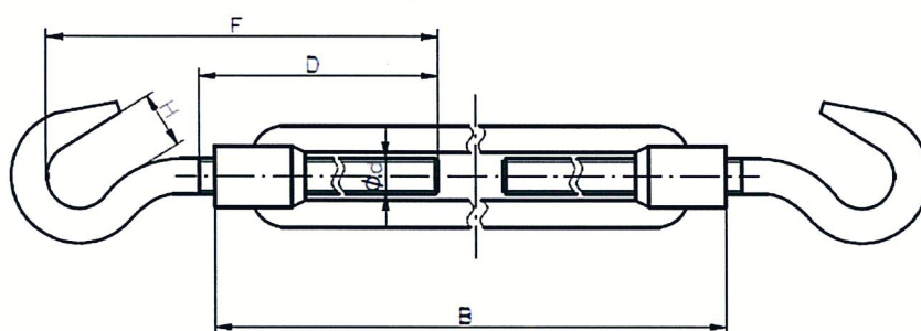
Rys. A1. Nakrętka napinająca rurowa SRM
