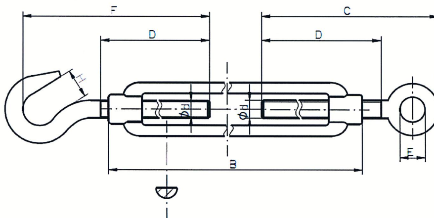
Rys. A7. Łącznik śrubowy dwustronny SRMI-HH
